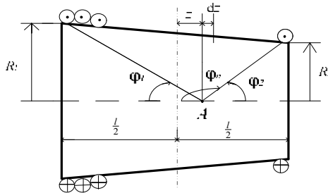
Рисунок 4 – К расчету напряженности магнитного поля конической однослойной катушки
