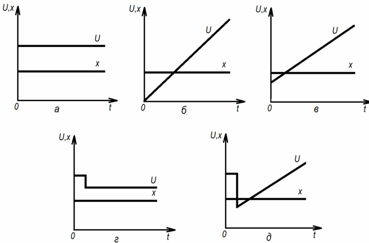
Рис. 3.4. Законы регулирования
