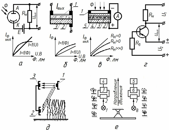
Рис. 4.18. Фотоэлектрические датчики
