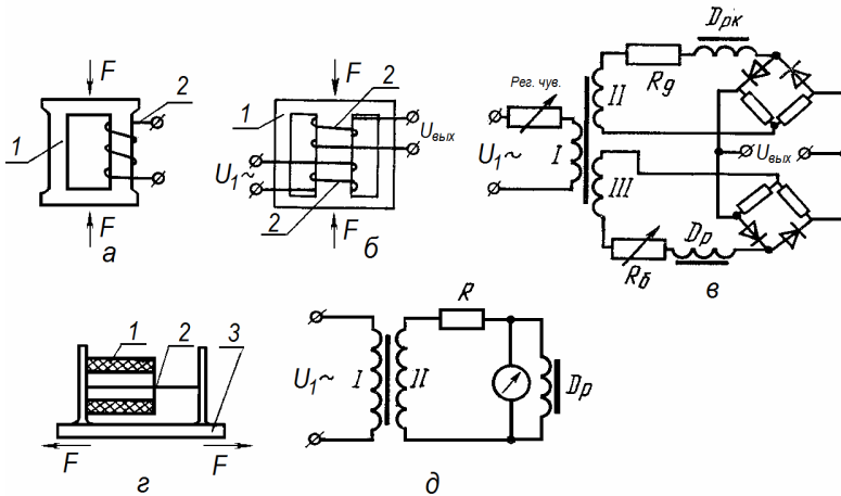
Рис. 4.12. Магнитоупругие датчики
