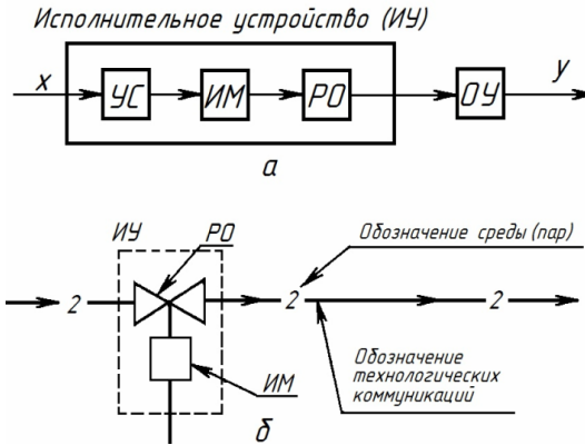
Рис. 4.31. Исполнительное устройство:
