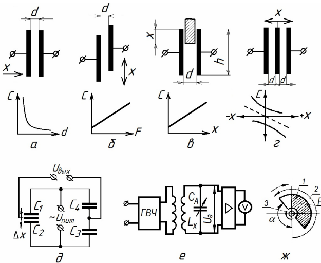
Рис. 4.17. Емкостные датчики
