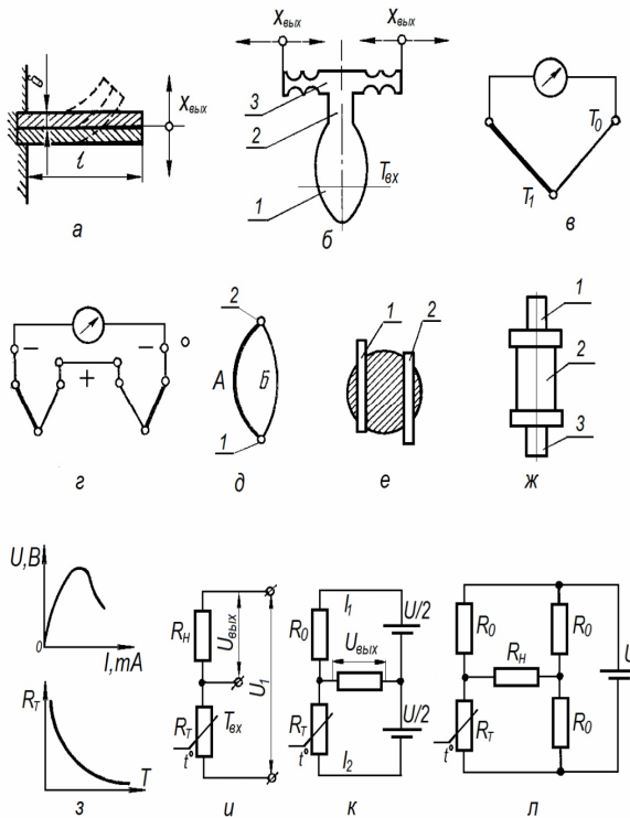
Рис. 4.20. Датчики температуры
