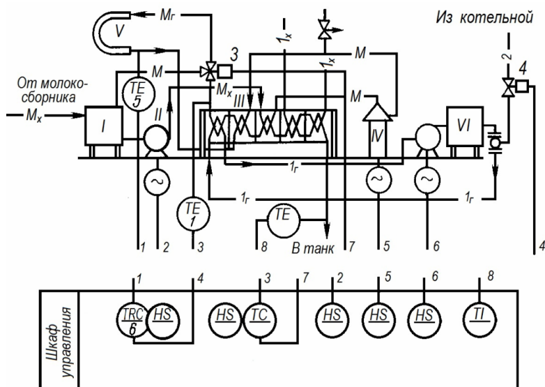
Рис. 6.3. Схема автоматизации установки ОПФ-1
