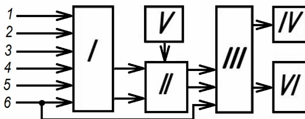
Рис. 5.13. Блок-схема системы контроля зерноуборочного комбайна
