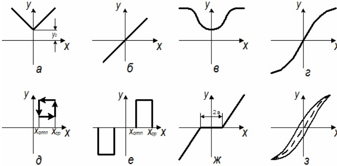
Рис. 4.1. Примеры статических характеристик элементов автоматики: а – линейная нереверсивная; б – линейная реверсивная; в – нелинейная нереверсивная; г – нелинейная реверсивная; д – релейная нереверсивная; е – релейная реверсивная; ж – с зоной нечувствительности (явление сухого трения); з – для ферромагнитных элементов
