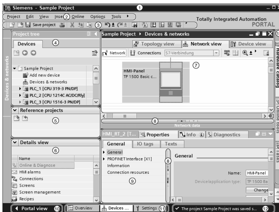
Рисунок 1 – Проектно-ориентированное представление структуры проекта (project view): 1 – панель заголовка (название проекта); 2 – главное меню; 3 – панель кнопок управления; 4 – дерево проекта; 5 – отображение других проектов, связанных с данным проектом; 6 – подробные данные об объекте, выбранном в дереве проекта; 7 – рабочая область окна; 8 – разделители; 9 – окно инспектора свойств объектов; 10 – переход к порталному представлению; 11 – панель переключения между задачами; 12 – строка состояния; 13 – панель вкладок библиотек компонентов
