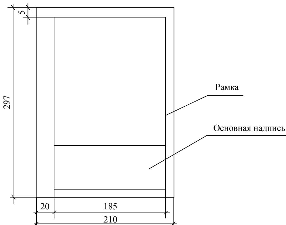
Рисунок 8 – Компонка и размеры листа текстовой части ПЗ
