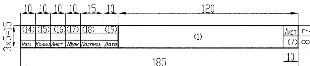
Рисунок 9 – Форма основной надписи для листов ПЗ
