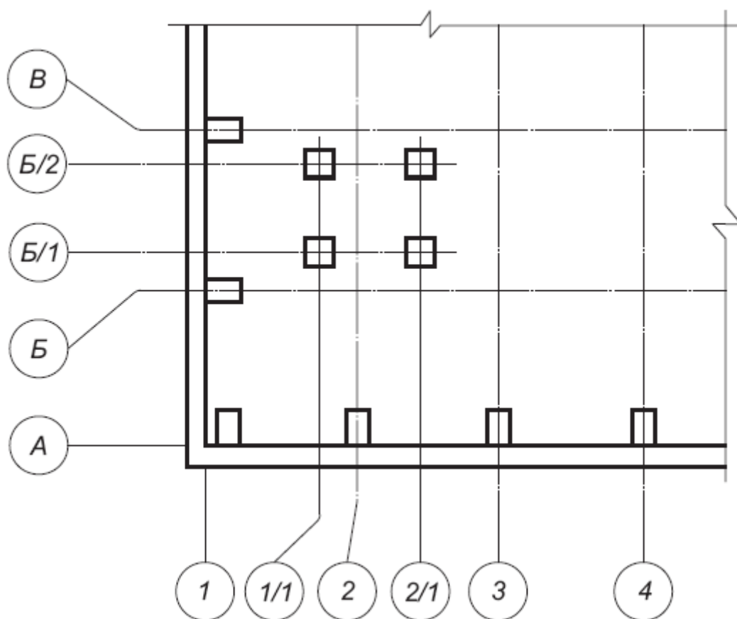
Рисунок 6.21 – Обозначение координационных осей
