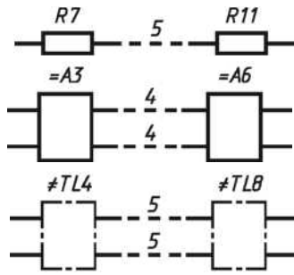
Рисунок 6.24 – Условные графические обозначения схем
