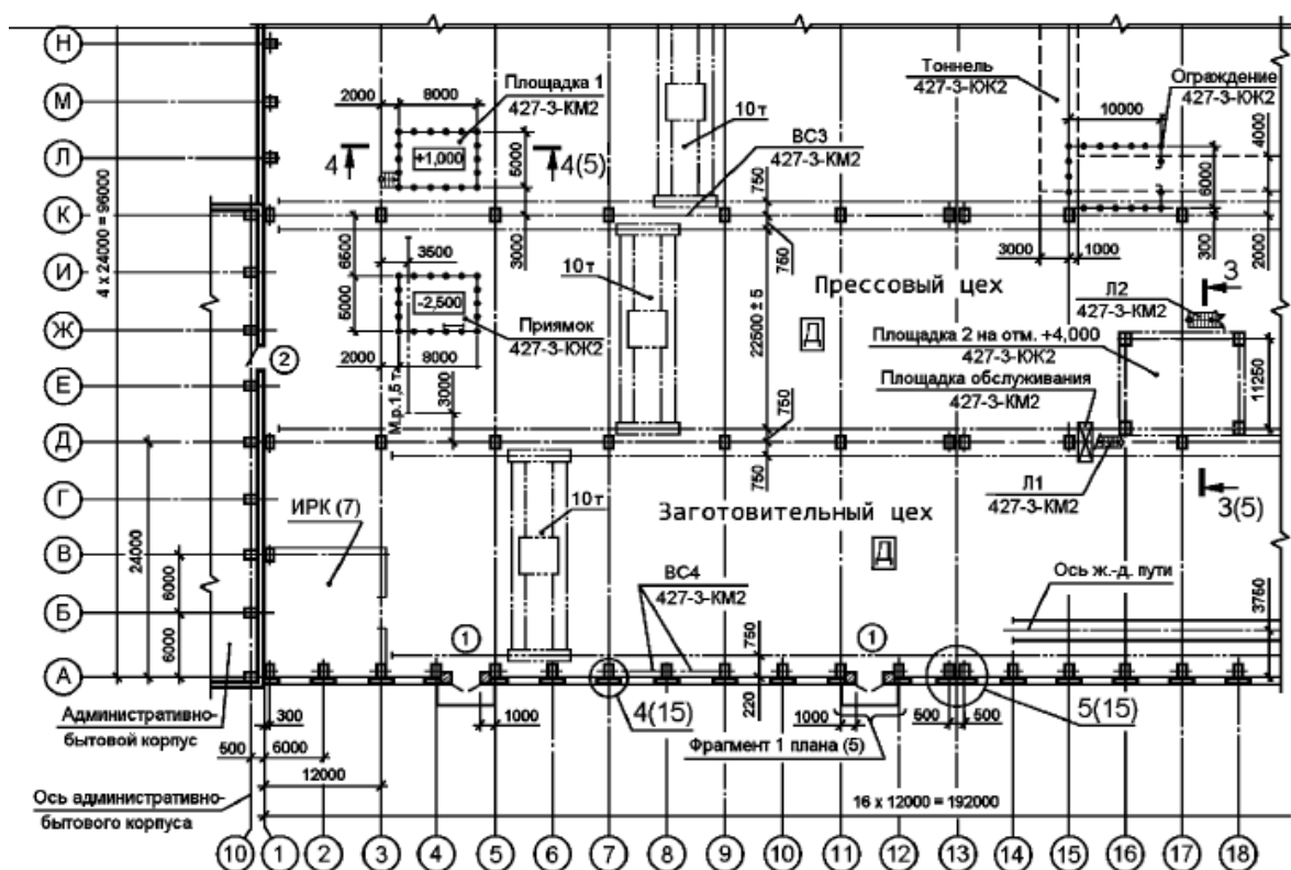
Рисунок X.1 – Пример выполнения плана одноэтажного производственного здания
