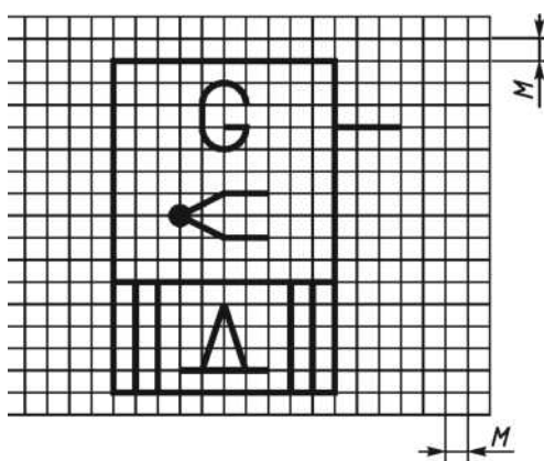
Рисунок 6.25 – Условное графическое изображение элементов
