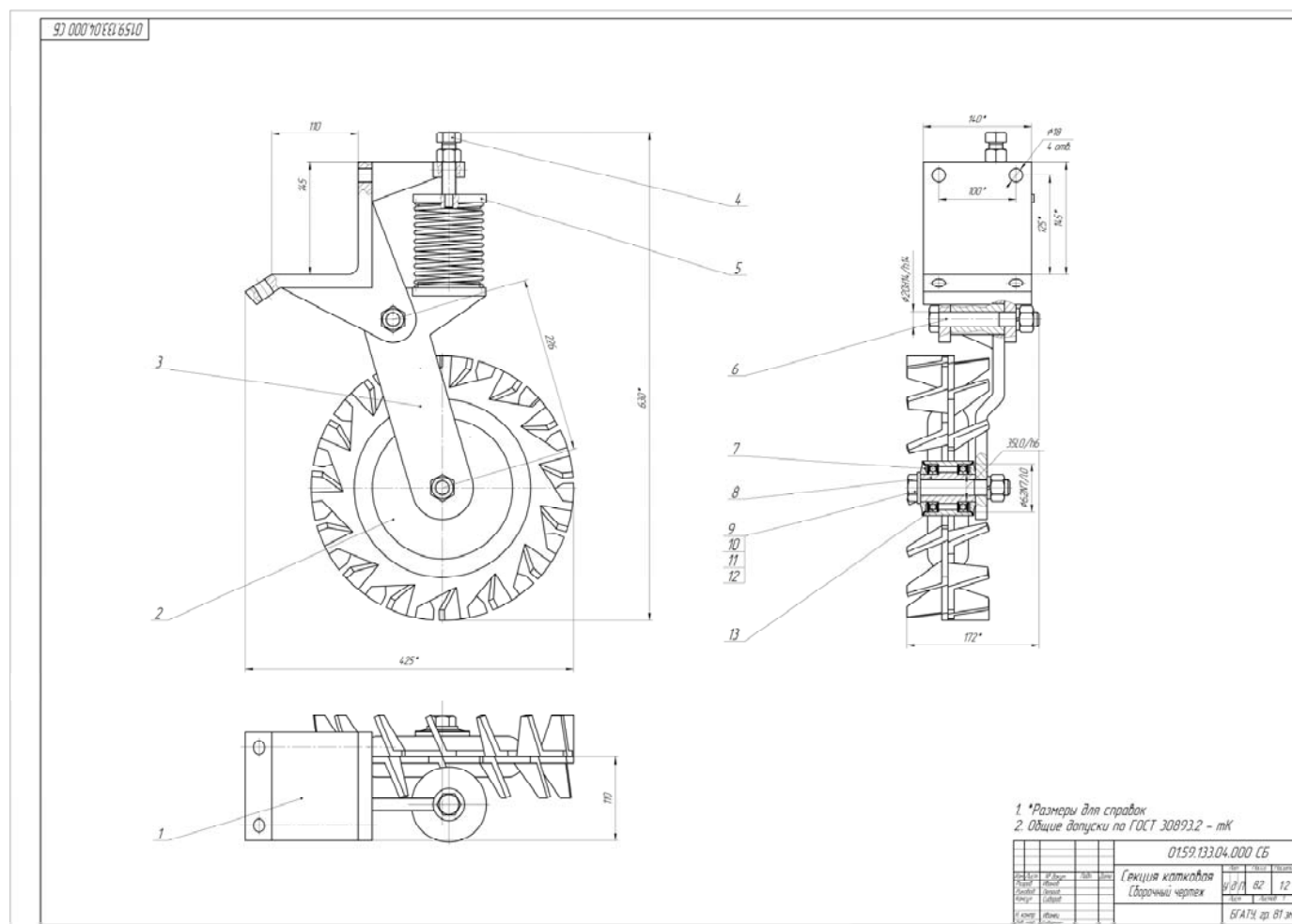
Рисунок Т.1 – Пример оформления сборочного чертежа
