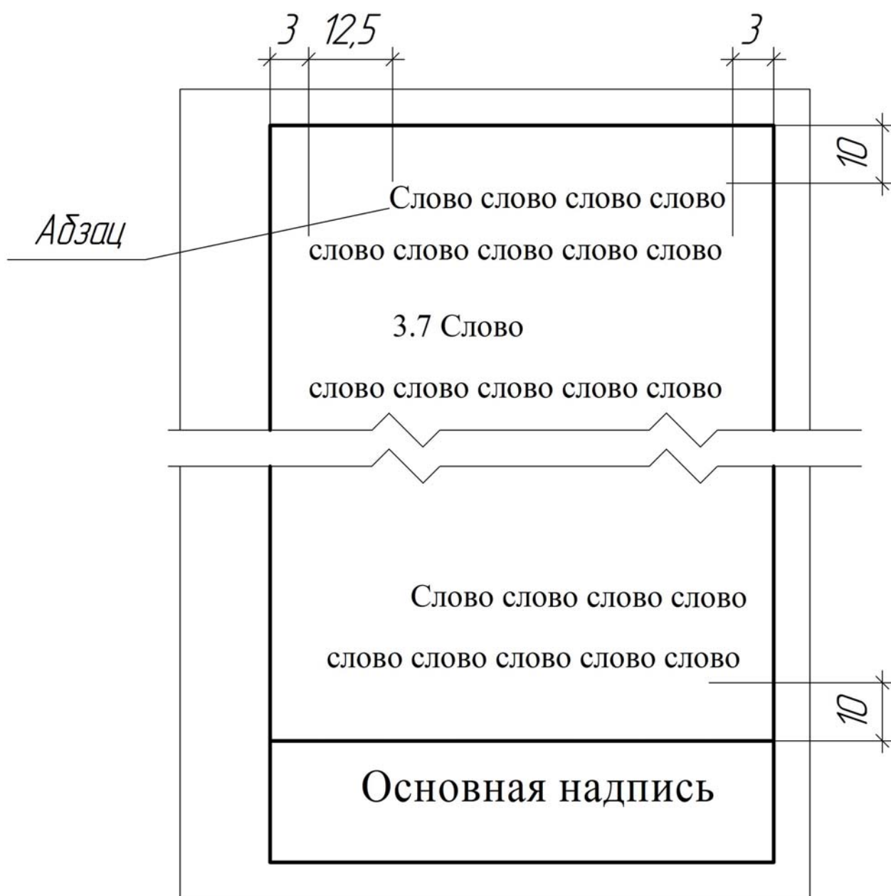
Рисунок 5.2 – Расположение текста на листе
