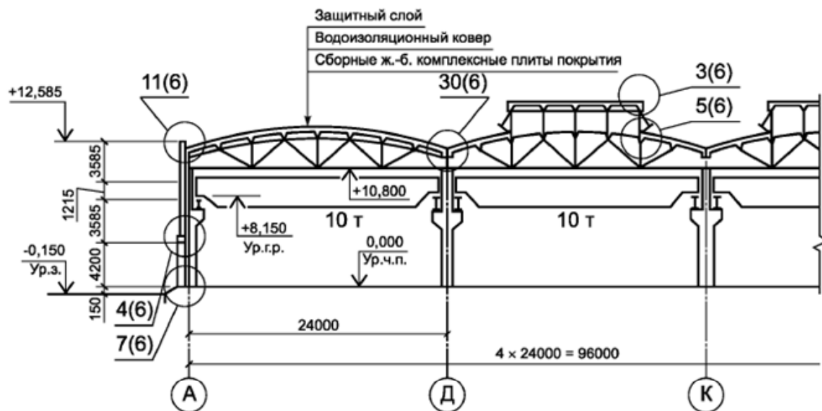
Разрез 1-1
