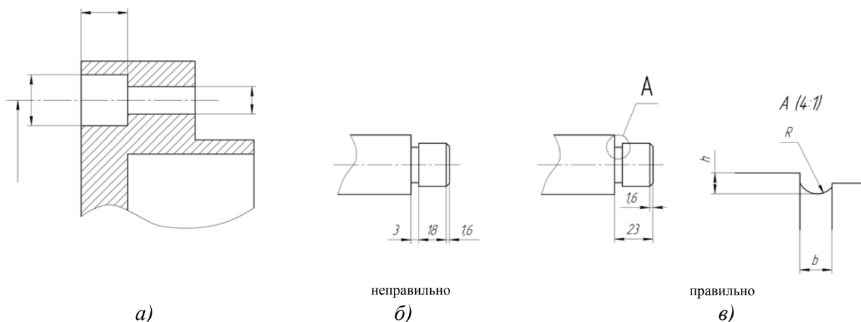
Рисунок 6.6 – Примеры нанесения размеров на чертежах
