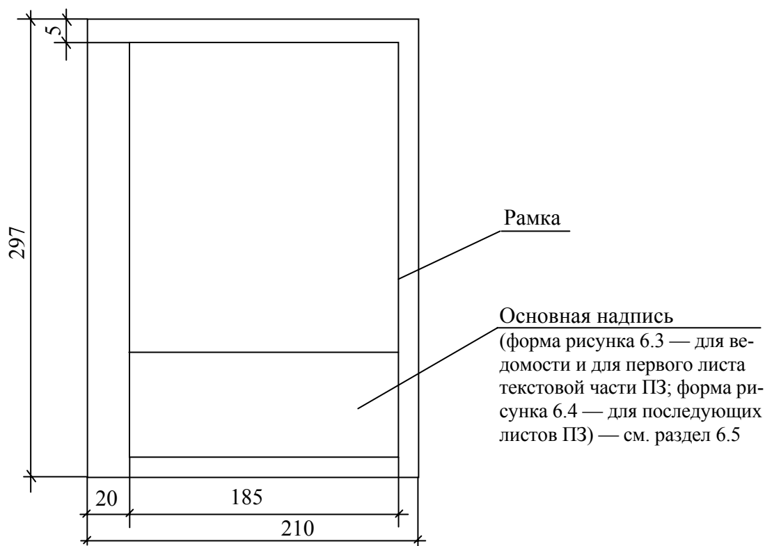
Рисунок 5.1 – Компоновка и размеры листа текстовой части ПЗ
