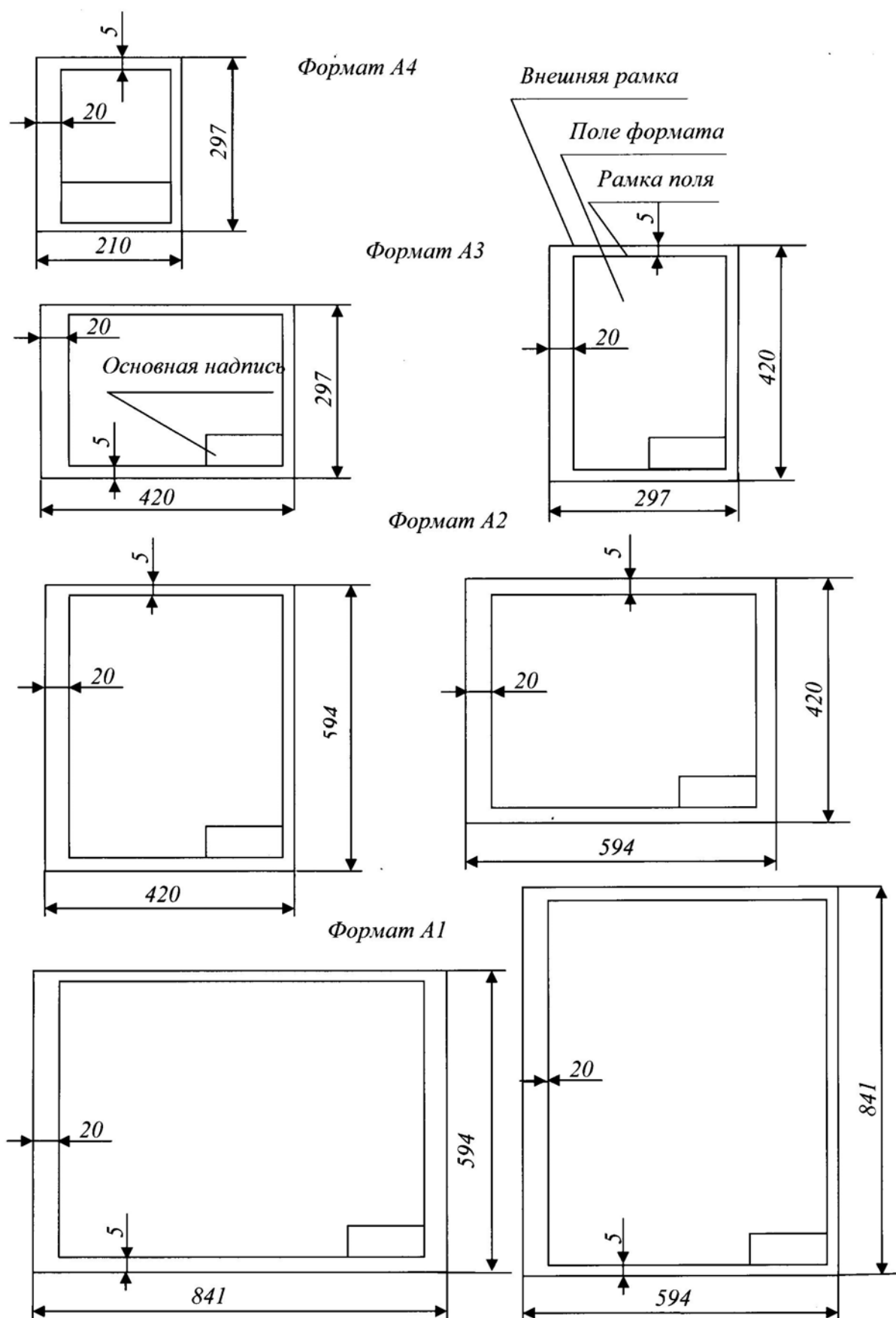
Рисунок 6.1 – Форматы листов
