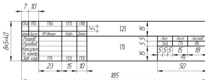
Рисунок 6.3 – Форма основной надписи, которая применяется для листа ПЗ, с которой начинается изложение текстовой части записки (обычно лист «Содержание»), ведомости комплекта проектной документации, спецификаций конструкторской разработки и оборудования
