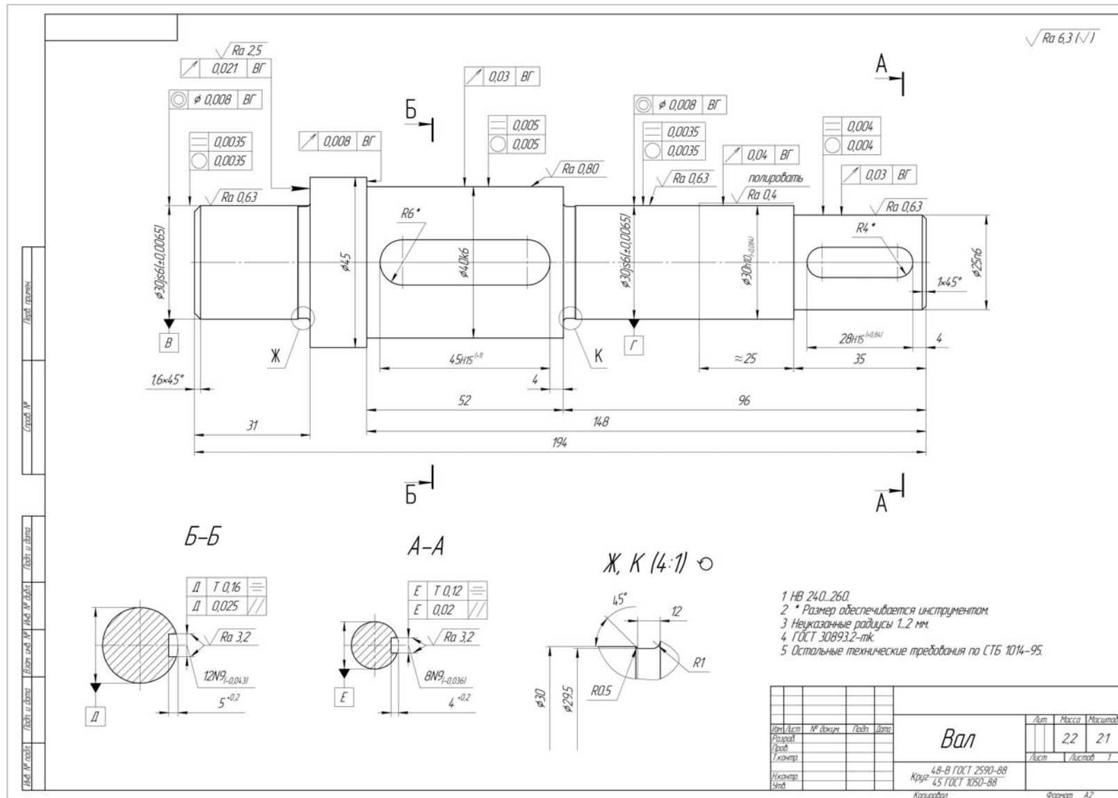
Рисунок 6.8 – Пример чертежа вала
