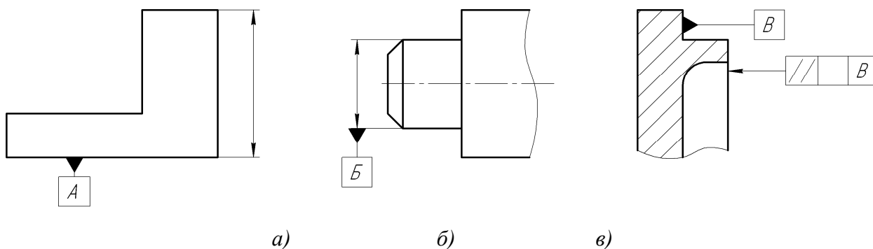
Рисунок 6.7 – Правила нанесения условных обозначений баз на чертежах деталей
