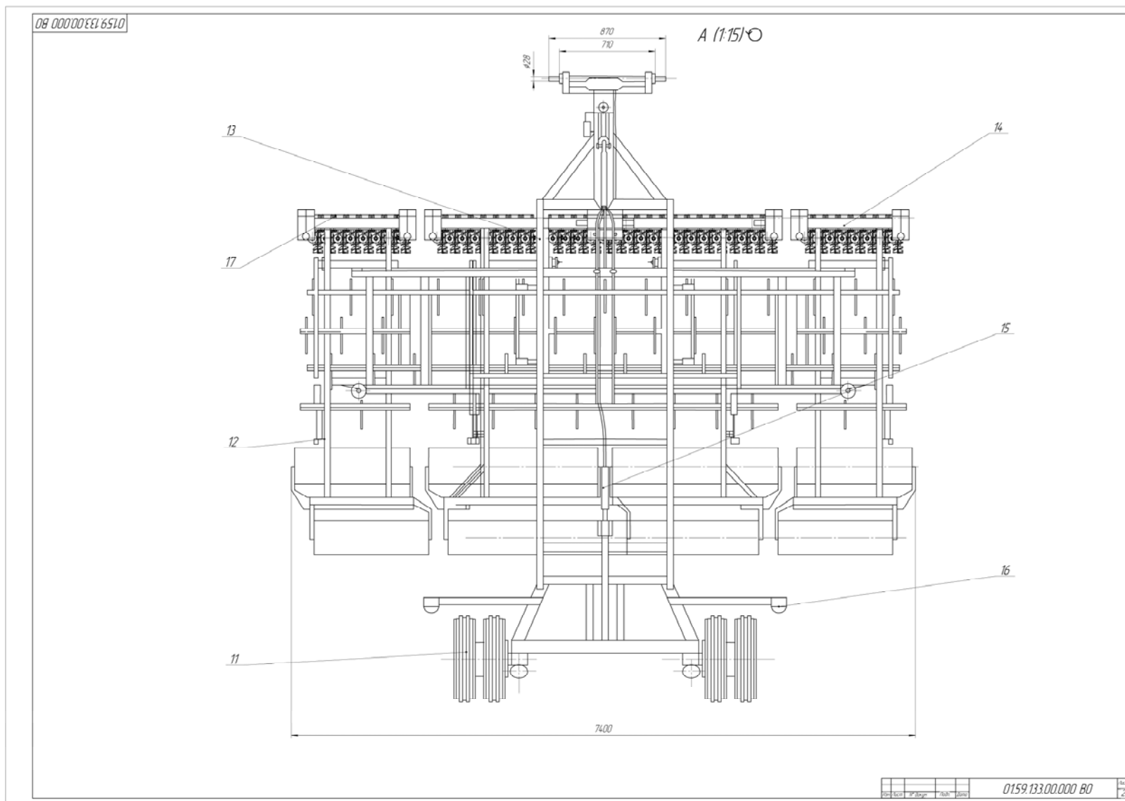
Рисунок С.2 – Пример оформления последующих листов чертежа общего вида
