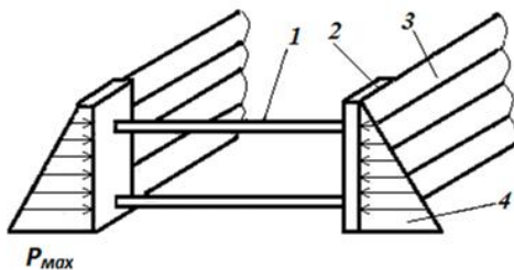
Рис. 10.3. Схема щитового крепления: 1 – распорки; 2 – стойки; 3 – щиты; 4 – эпюра давления
