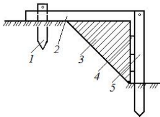
Рис. 10.5. Анкерное крепление траншеи:
