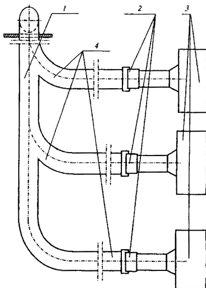
Рис. 7.3. Схема установки на группе оборудования комбинированных взрыворазрядных устройств, объединенных коллектором: 1 – коллектор; 2 – комбинированные или клапанные взрыворазрядные устройства; 3 – защищаемое оборудование; 4 – отводящие трубопроводы
