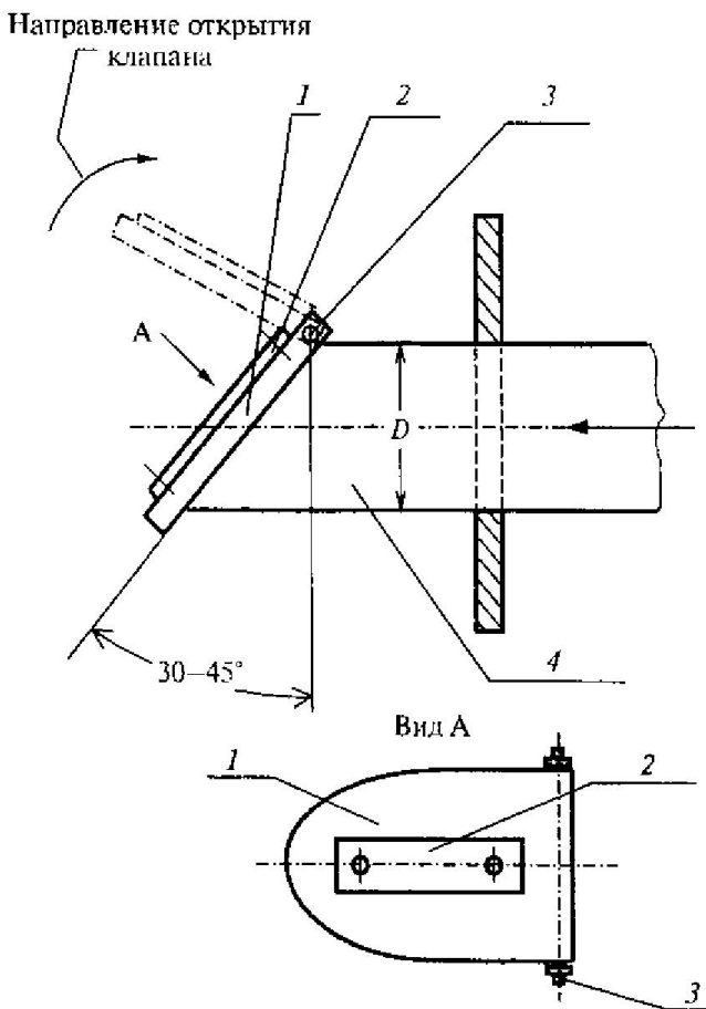
Рис. 7.2. Конструктивная схема взрыворазрядного устройства с откидным клапаном и горизонтальным отводящим трубопроводом: 1 – крышка откидная; 2 – груз; 3 – ось поворота крышки; 4 – соединяющий (входной) патрубок
