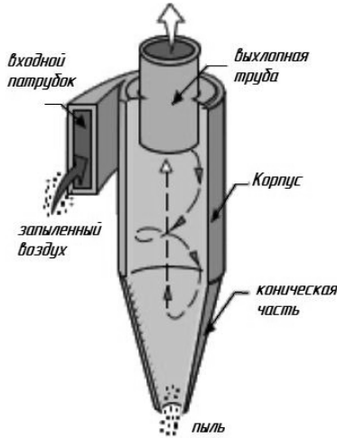
Рис. 8.3. Циклон
