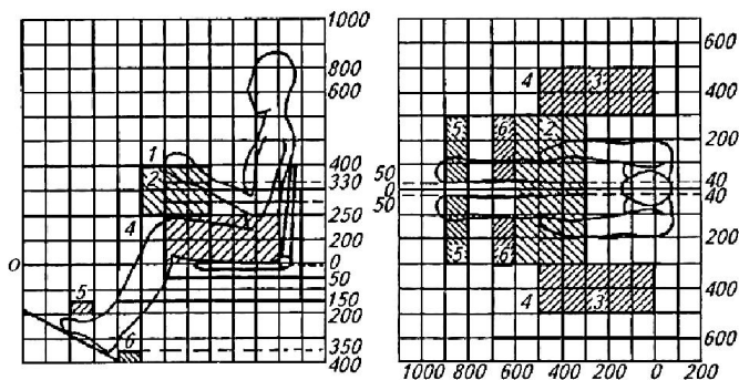
Рис. 3.1. Зоны расположения органов управления трактором: 1 – нижняя точка рулевого колеса; 2 – центры рукояток рычагов механизма поворота и рычагов, установленных на рулевой колонке и передней панели; 3, 4 – предпочтительные и допустимые зоны расположения других рычагов; 5, 6 – центры и нижние кромки опорных площадок педалей, приводимых в действие ногами
