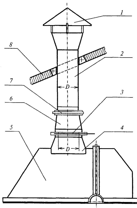
Рис. 7.1. Схема расположения на головке нории взрыворазрядного устройства шибераго типа:
